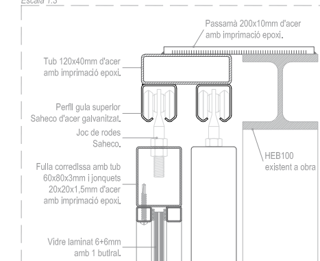
Detall horitzontal (porta tancada) Escala 1:3
