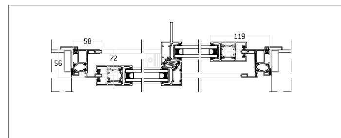
Secció Horitzontal [E 1:4]: Corredissa 2F-2V
