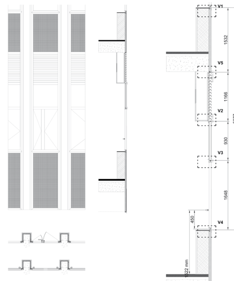
SECCIÓN VERTICAL
