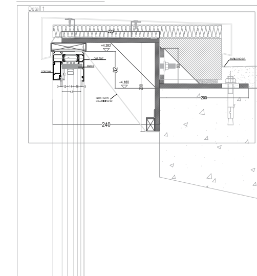
SECCIO VERTICAL
