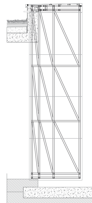
SECCIÓ VERTICAL (1)
