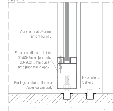
Detall inferior per fulla corredissa Escala 1:3
