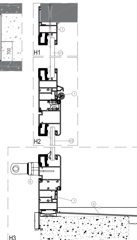
DETALLES SECCIÓN 1
