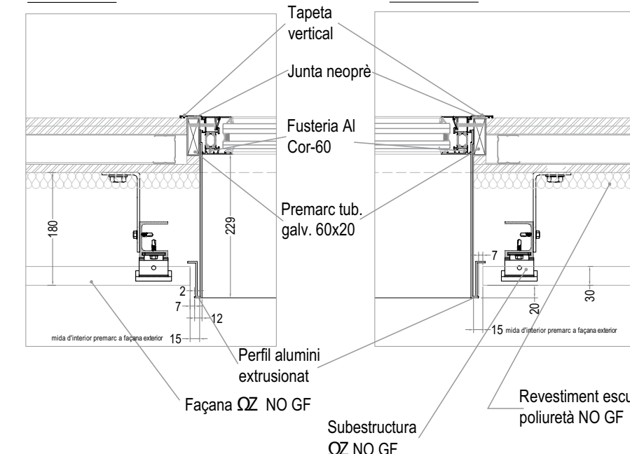
DETALL C
