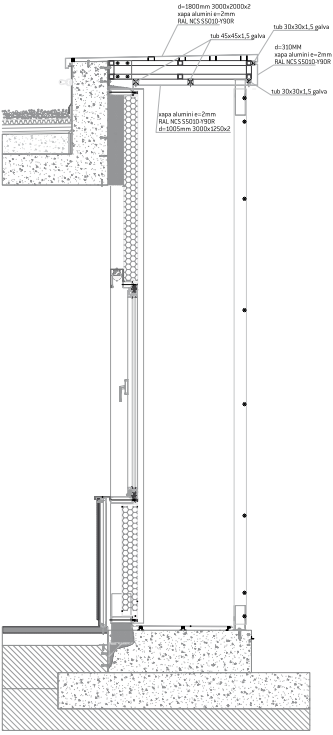
SECCIÓ VERTICAL (2)
